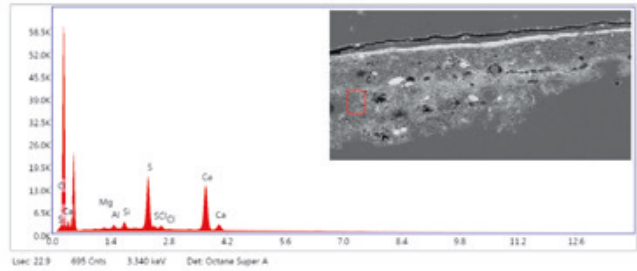
Figura 15: Análisis de elementos químicos mediante EDS de la muestra AMSA-P-02-2023. Estrato 1 con presencia de magnesio, aluminio, silicio, azufre, cloro, calcio y su espectro.
